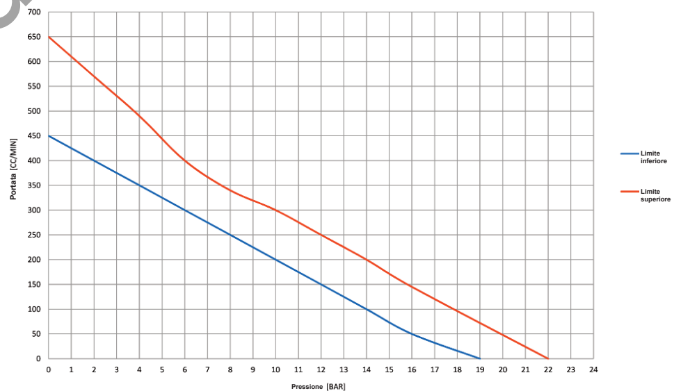
Curva delle prestazioni
